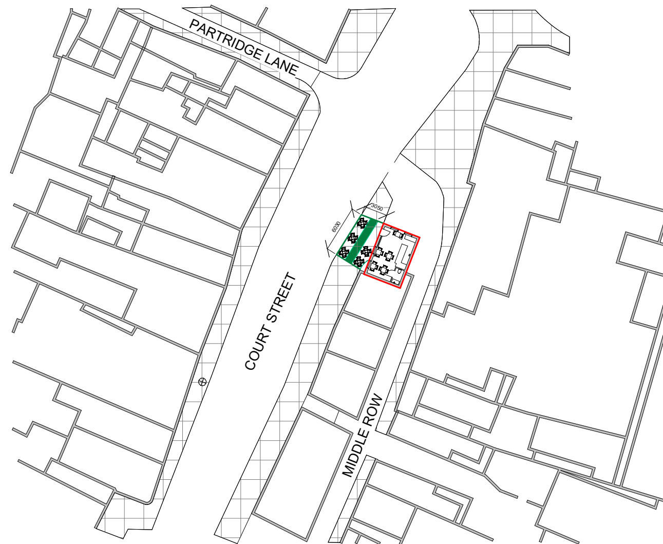
1 SITE PLAN 1:500
